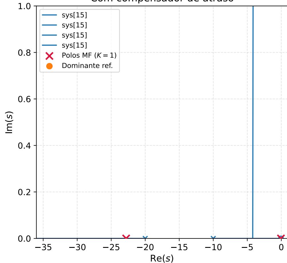
Com compensador de atraso
